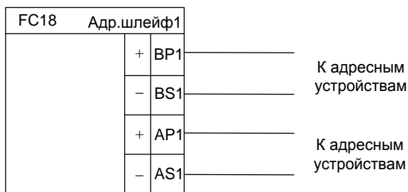
Рис. Схема подключения адресного шлейфа (шлейф 2 подключается аналогично)
